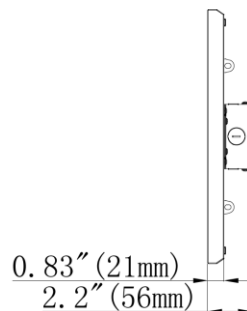
PHB-III-2-110W Dimensions mm | 605(L) x 320(W) x 56(D) inch | 23.8(L) x 12.6(W) x 2.2(D)
