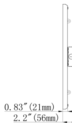
PHB-III-2-165W/ PHB-III-2-220W Dimensions mm | 605(L) x 440(W) x 56(D) inch | 23.8(L) x 17.3(W) x 2.2(D)
